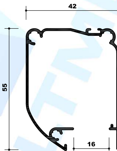
HY2803-37 CABEZAL P42
