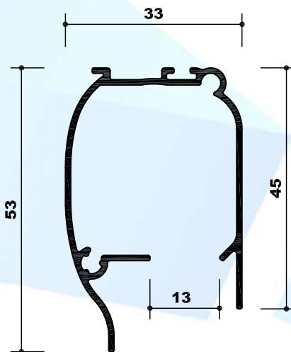
HY2504-37 CABEZAL R33
