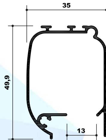
HX1989-37 CABEZAL R35
