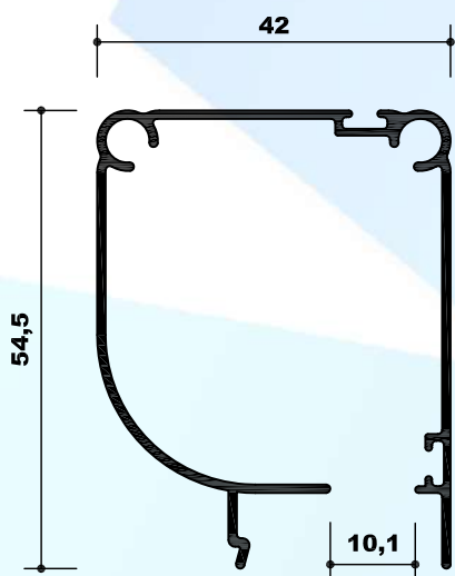
HY2571-37 CABEZAL R42
