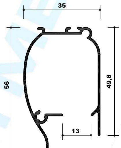
HY2570-37 CABEZAL R35
