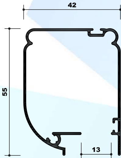
HX1988-37 CABEZAL P42
