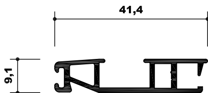
HX1992-37 TIRADOR MOSQUITERA
