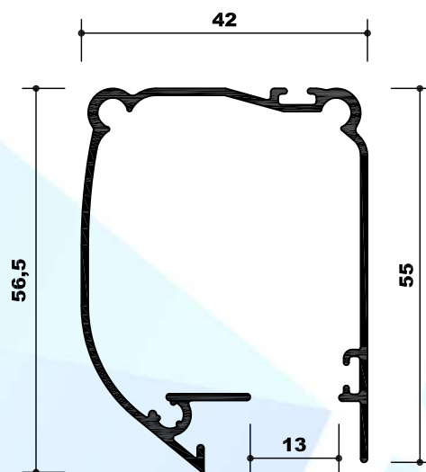
HY2572-37 CABEZAL P42
