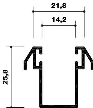
10277 GUIA EMBUTIR CON ALA
