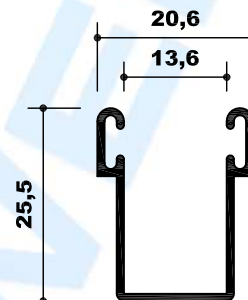
00748 GUIA DE EMBUTIR
