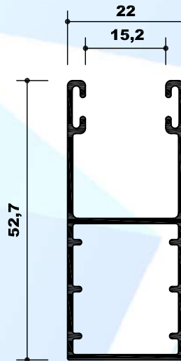
10036 GUIA 52,7x22 - H 25
