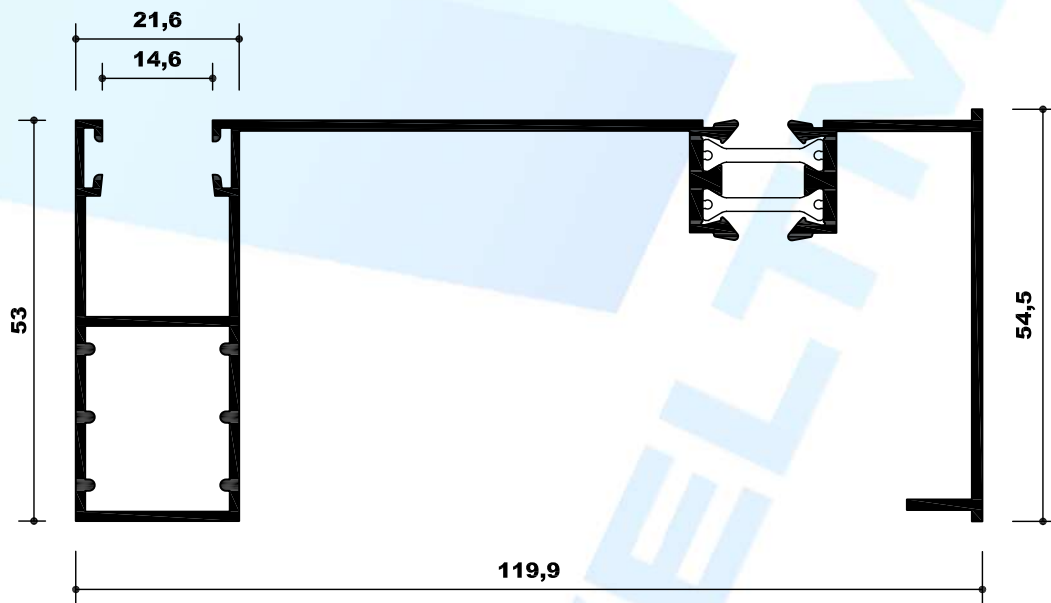
A-1887 GUIA ROTURA 120mm
