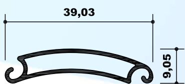
1442A LAMA AUTOBLOCANTE
