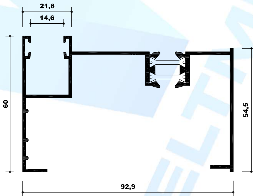
16135 GUIA ROTURA 93mm
